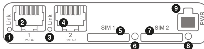
Рис. 2. Вид спереди R11-A.Wn
